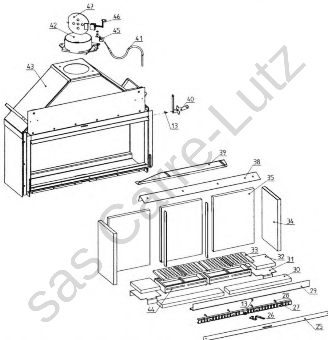
Vue éclatée de la chambre de combustion
